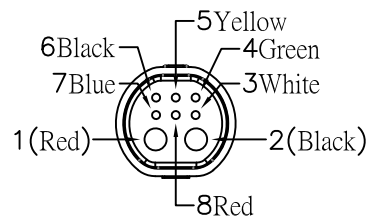
WPB25-26F 2+6
