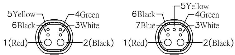
WPB25-24F 2+4
