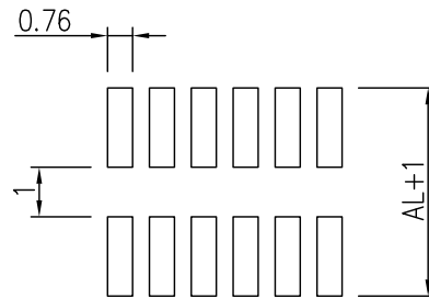
P.C.Board Layout
